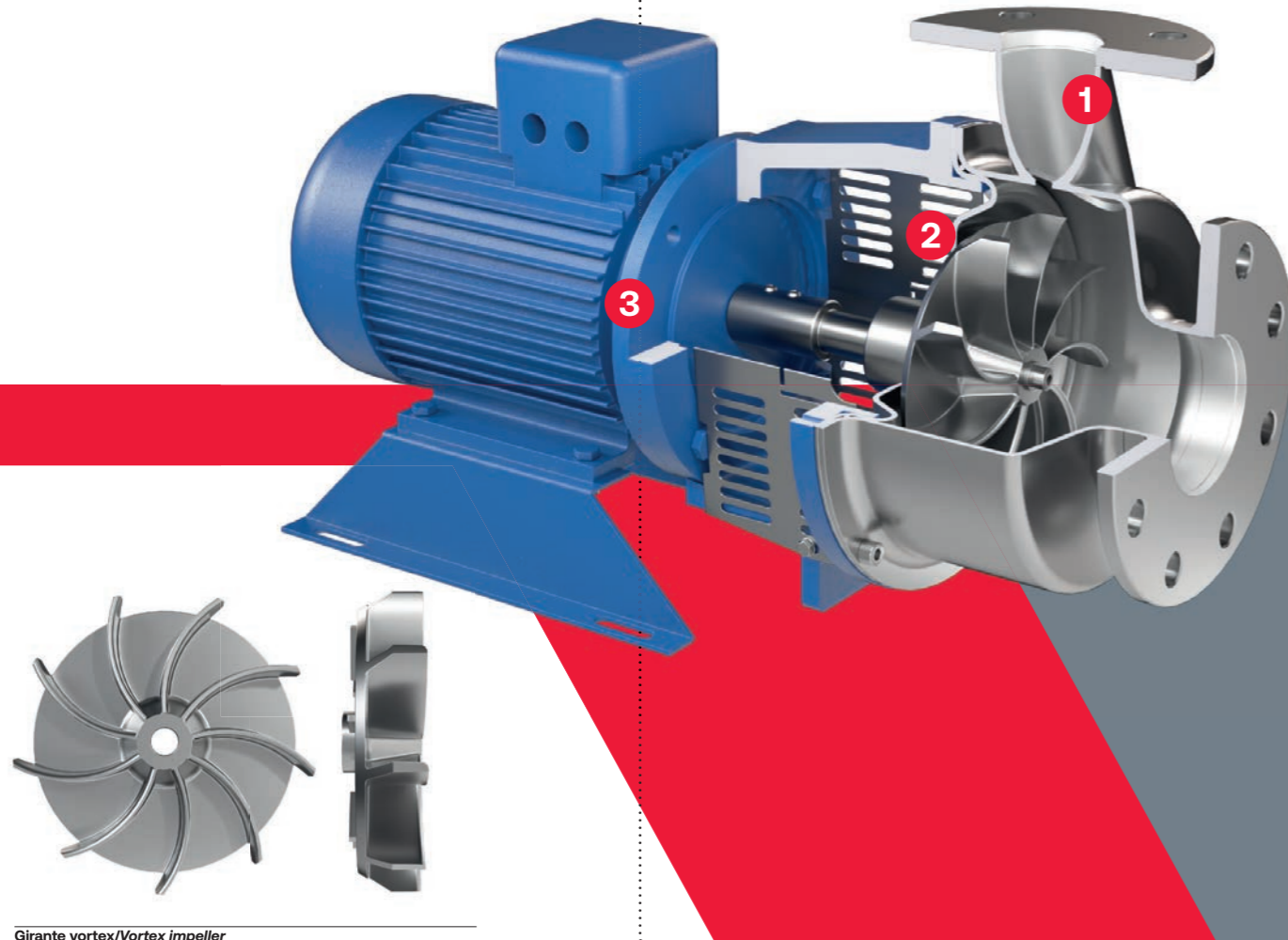
Girante vortex/Vortex impeller
