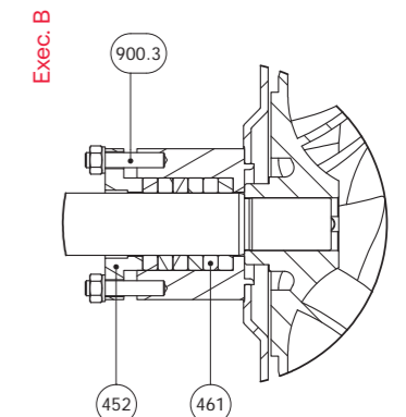
Tenuta a baderna Packing gland
