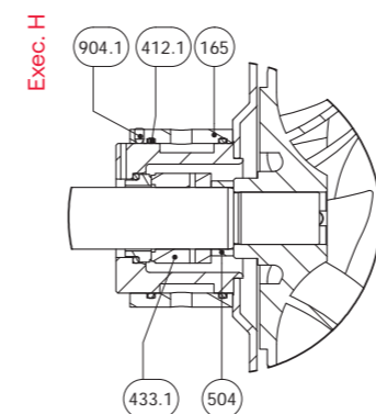
Camera riscaldamento/raffreddamento Cooling/heating jacket
